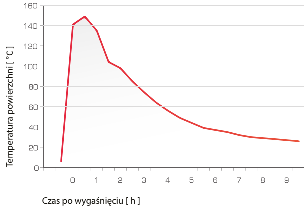
Piecyk kominkowy z akumulacją
